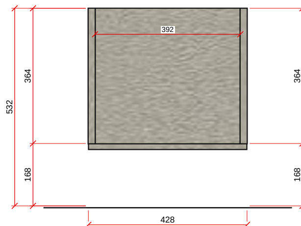
PAINEL - ESC. 1:10
