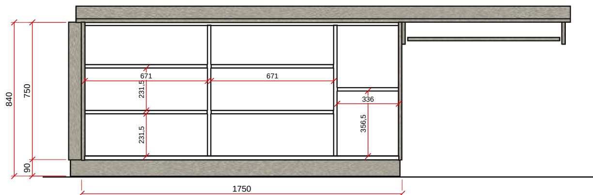
VISTA A - ESC. 1:20
